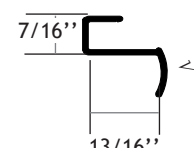
Door Pull
